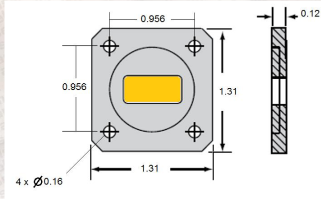
Şekil 1. Teknik çizim. Boyutlar inç cinsindedir. Konum ve çap toleransları 0.012 inç'tir.
